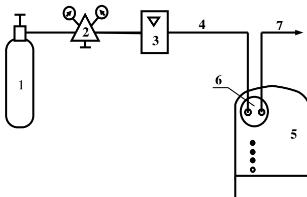
Рисунок Е.1 – Установка насадки для подачи ПГС
